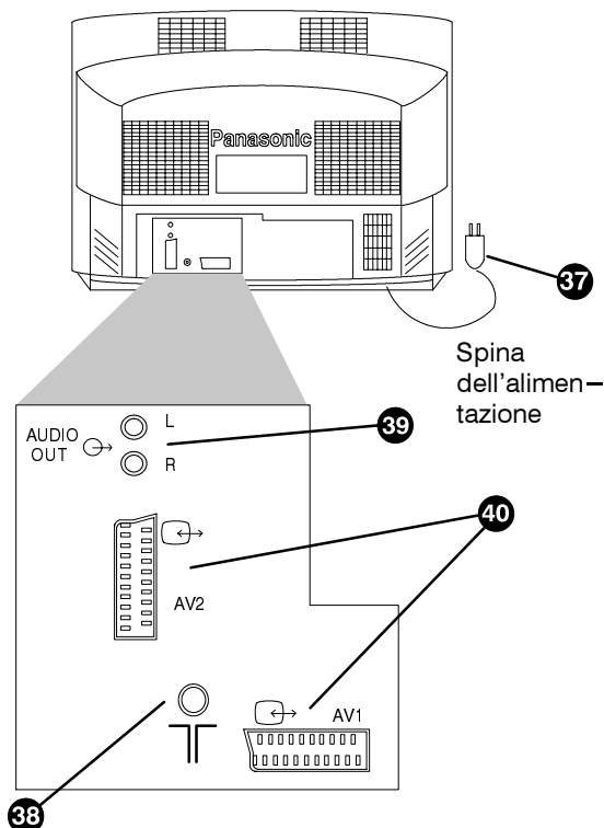
40 Terminale SCART a 21 pin
